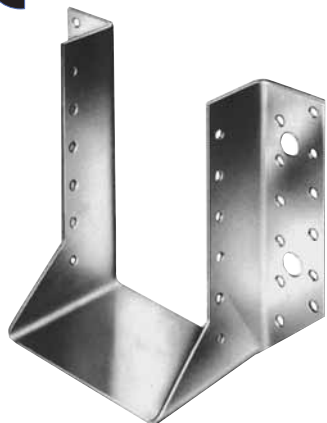
100×140 udadvendte flige
