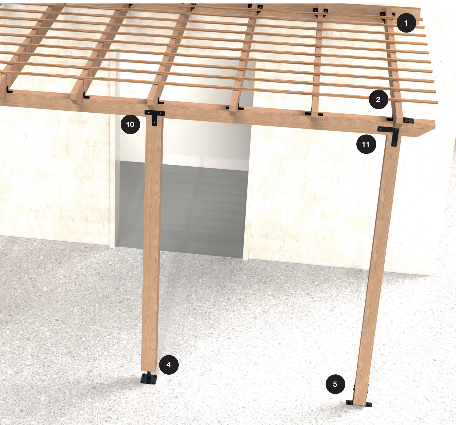
9 Stolpehætte
