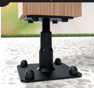
4 Justerbar søjlesko
